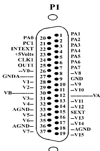
β Brochage du connecteur mâles de liaison Sub-D 37 points
