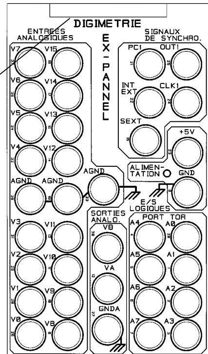
Implantation des douilles bananes carte EX-PANNEL
